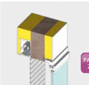
VOLET OUVERTURE SOUS-FACE
