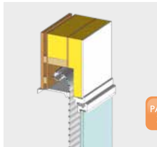
VOLET ROULANT POUR OSSATURE BOIS
