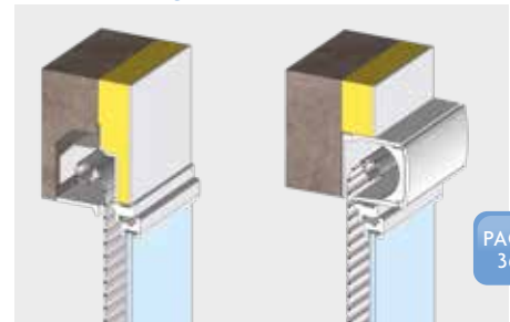
VOLET ROULANT 1/2 LINTEAU INCORPORÉ À LA MENUISERIE
