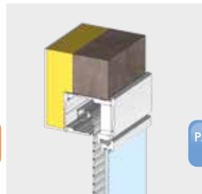
VOLET ROULANT INTÉGRÉ ENROULEMENT EXTÉRIEUR
